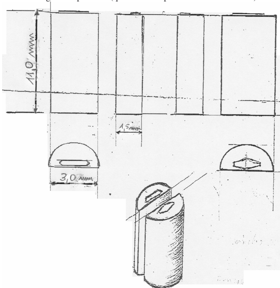
Disegno dei punzoni (quotato ed espresso in decimi di mm)
