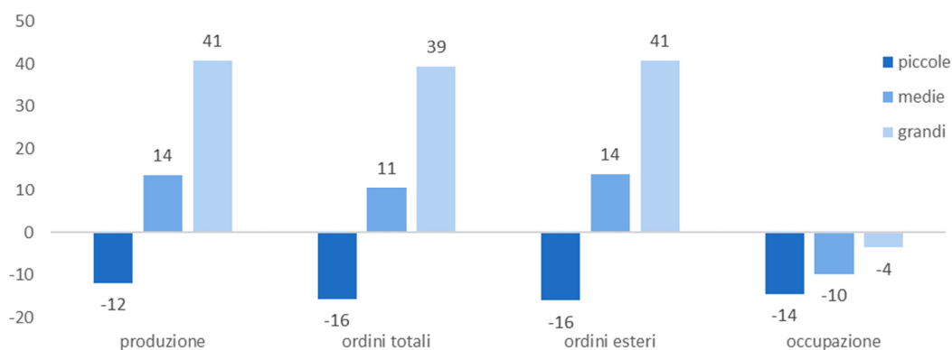
Graf. 2 – Previsioni: saldi ottimisti/pessimisti per dimensione di impresa
